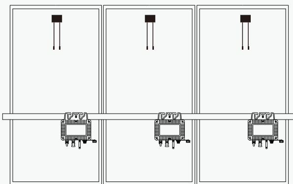
图1 微型逆变器安装位置
